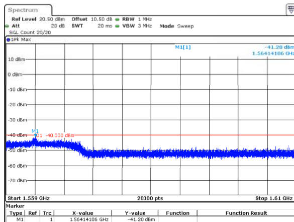
10MHz_Middle_QPSK_50@0(1559MHz~1610MHz)
