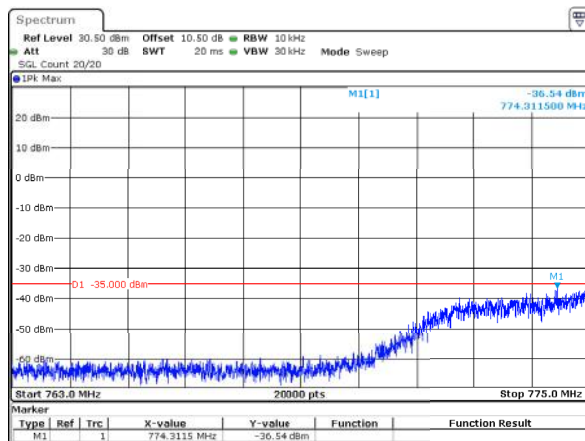
10MHz_Middle_QPSK_50@0(763MHz~775MHz)
