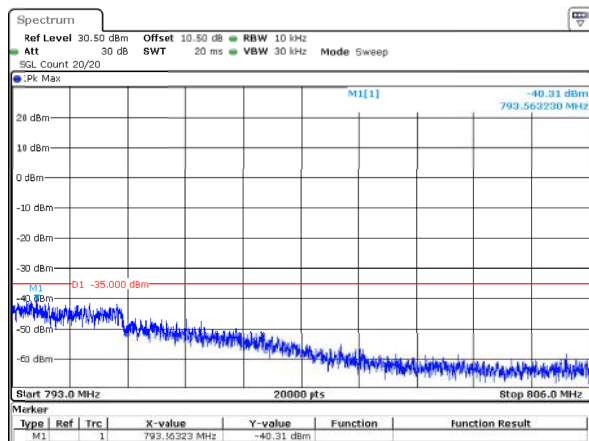
10MHz_Middle_QPSK_50@0(793MHz~806MHz)
