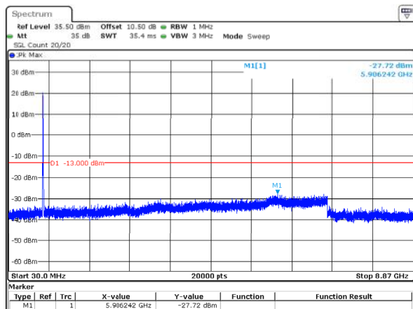
10MHz_Middle_QPSK_50@0(30MHz~8.87GHz)
