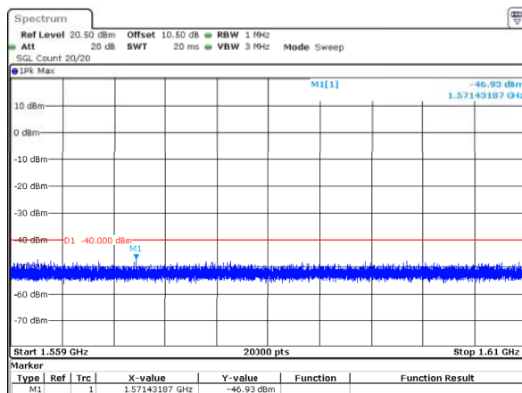
10MHz_Middle_QPSK_1@0(1559MHz~1610MHz)
