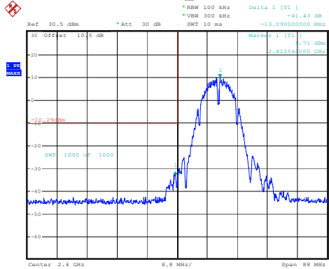
802.11b_2412MHz
