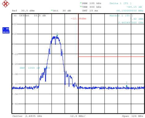
802.11b_2462MHz
