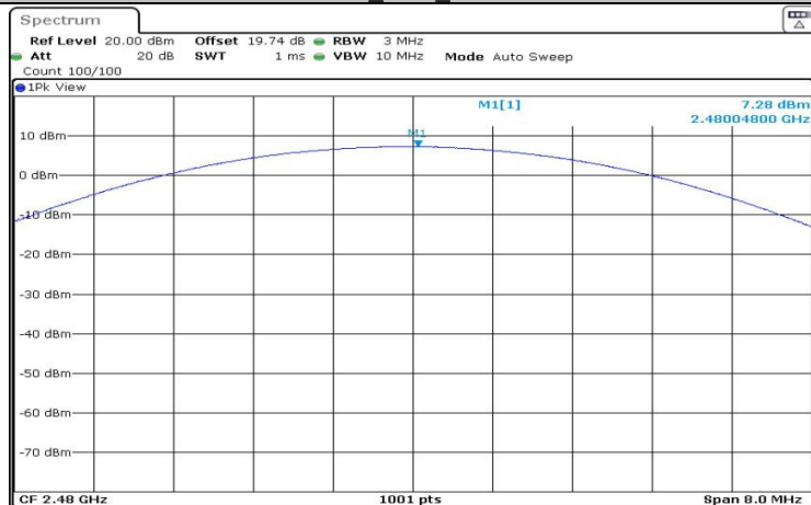
DH1_Ant1_2480
