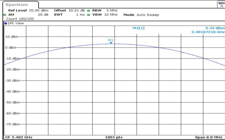
DH1_Ant1_2402
