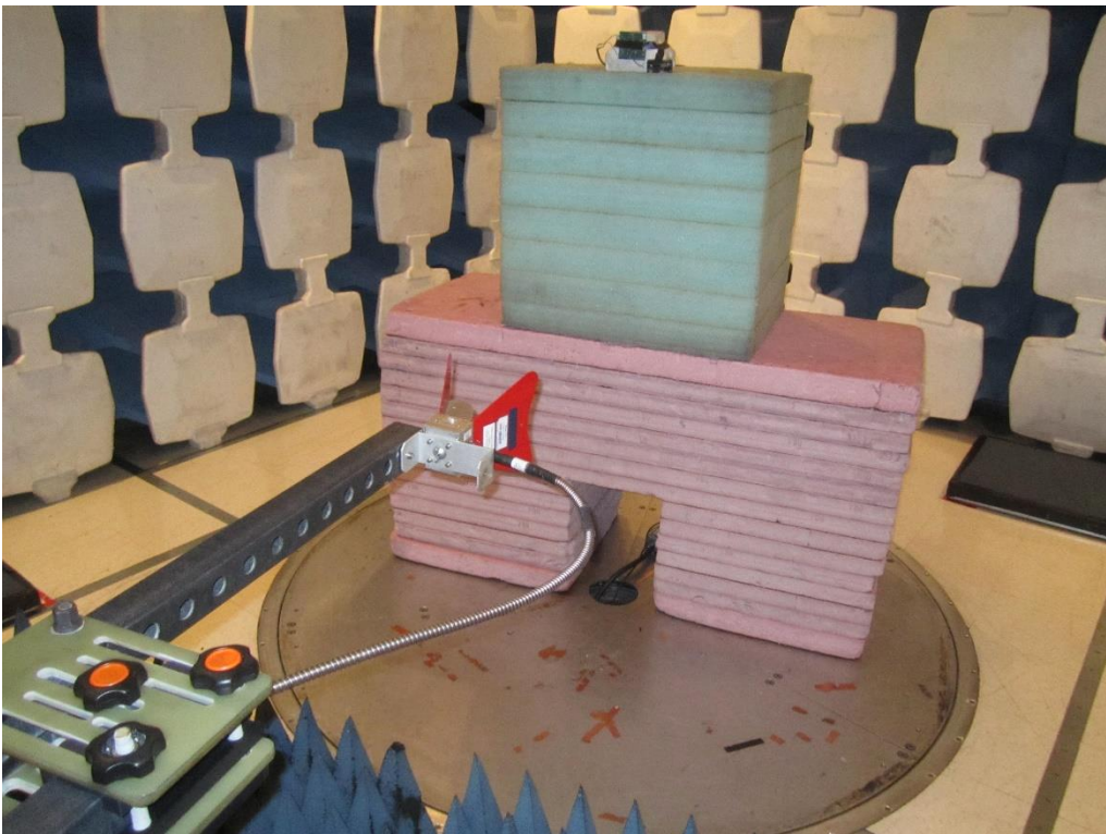
6-18GHz
