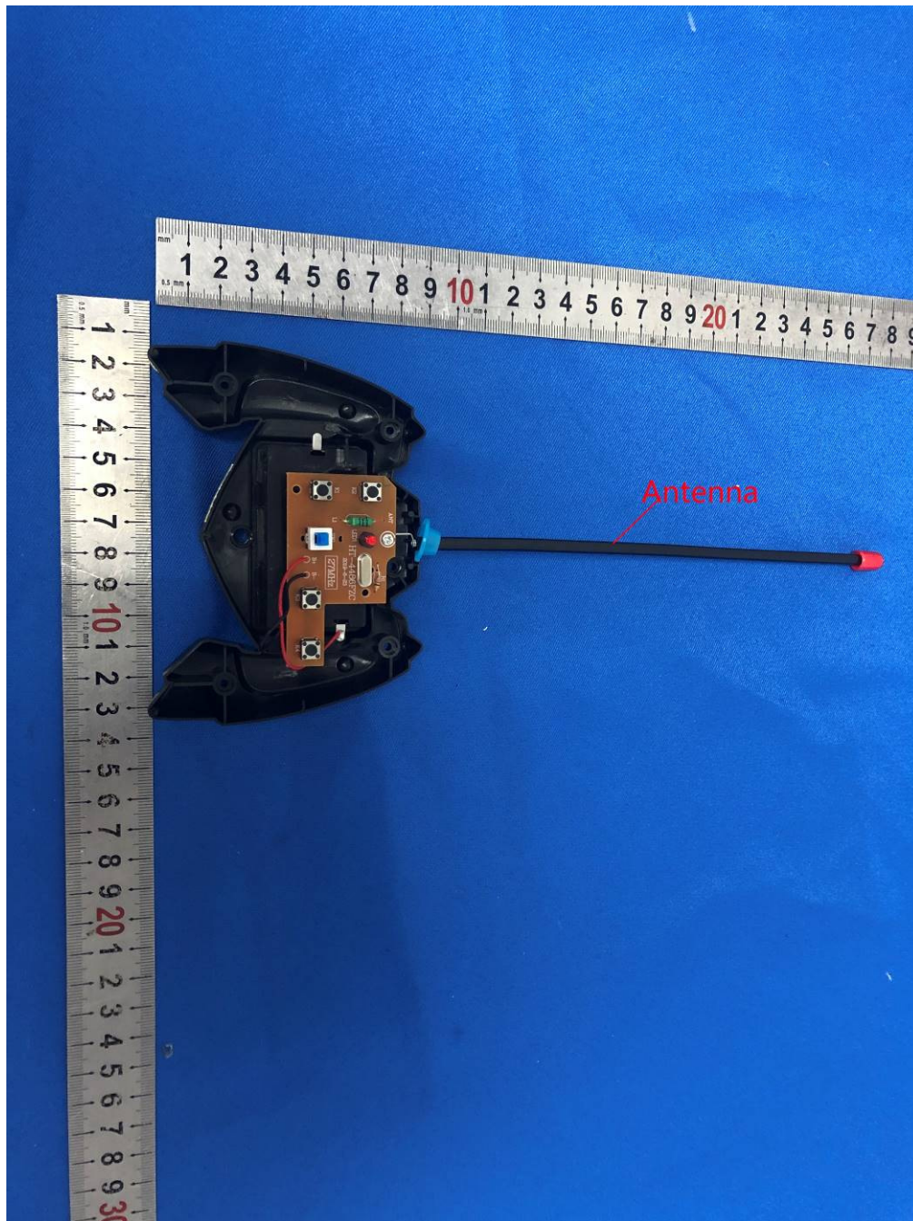
Antenna
