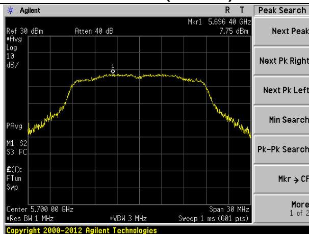
Channel 140 (5700MHz)
