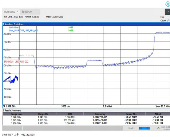
Band2_20MHz_QPSK_18700_1RB#99
