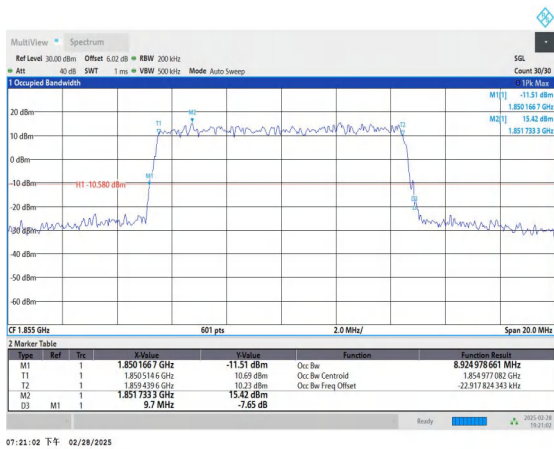
Band2-10MHz-QPSK-18650-50RB#0-PASS
