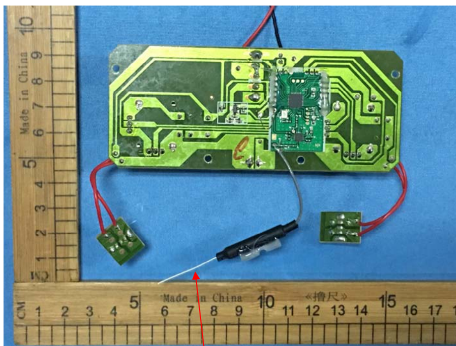
2.4G Antenna
