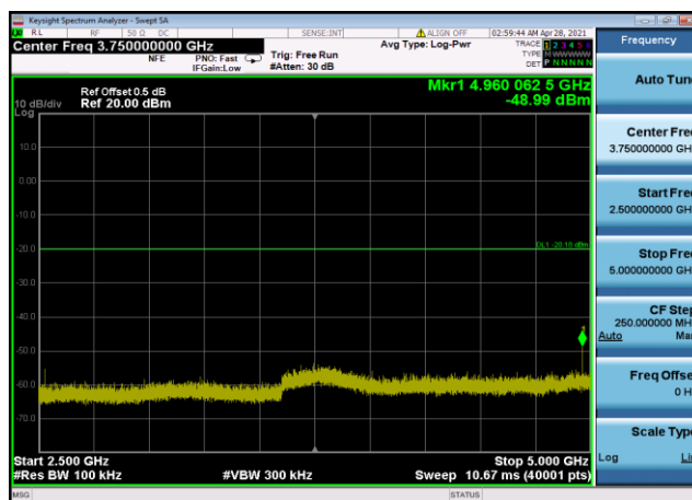
2480MHz,Plot 4,2500MHz~5000MHz
