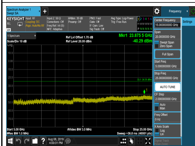
2480MHz,Plot 5,5000MHz~25000MHz
