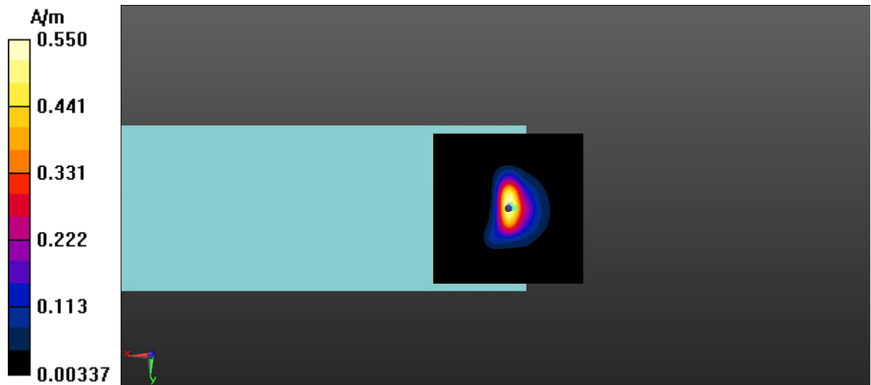
Fig A.1 T-Coil GSM 850-Z
