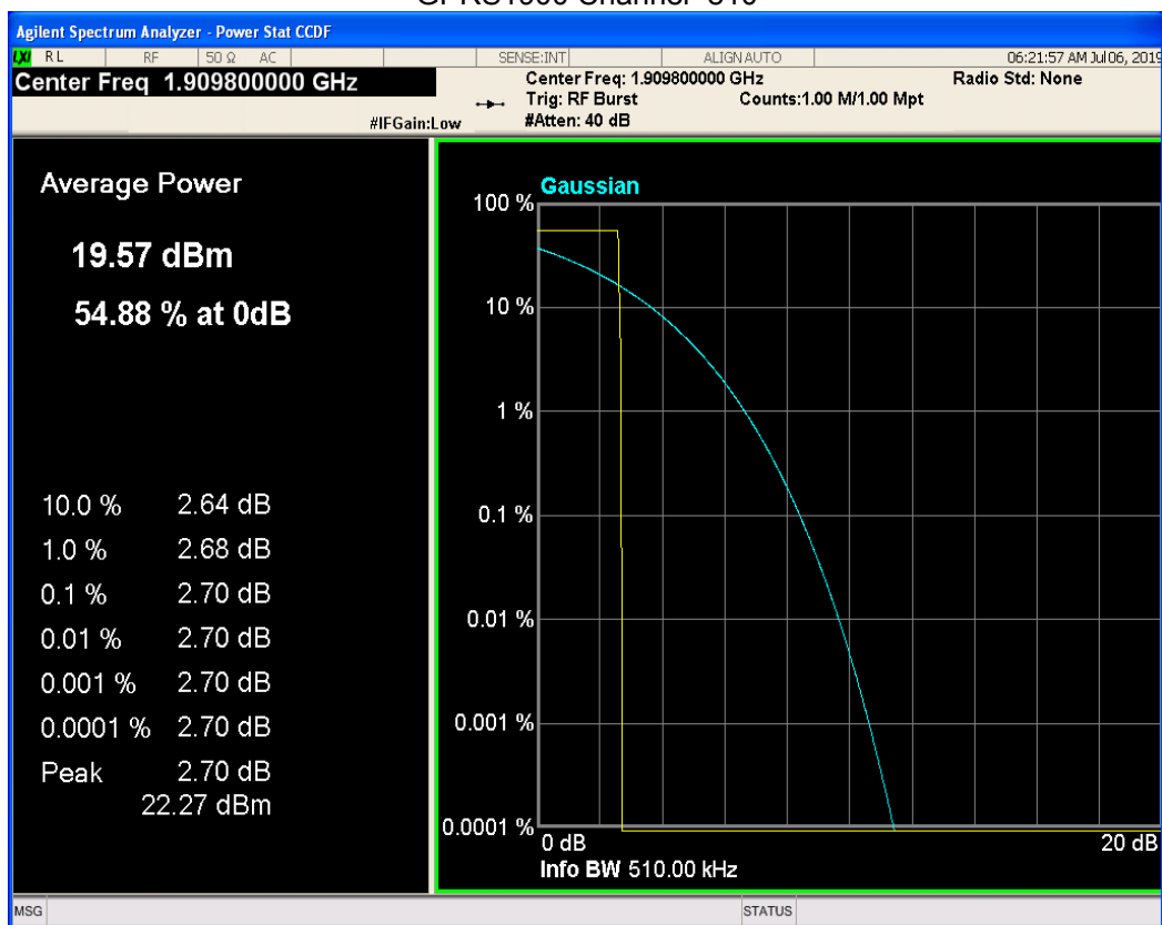
GPRS1900 Channel=810
