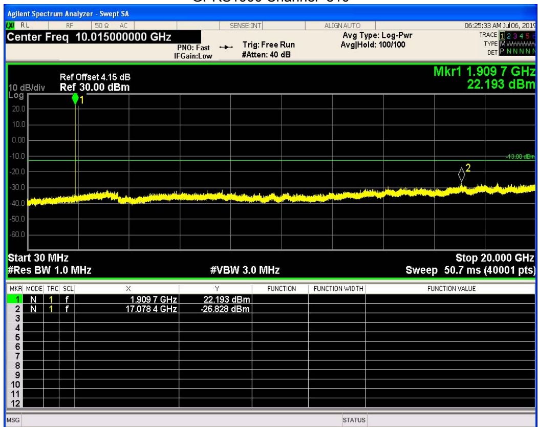
GPRS1900 Channel=810
