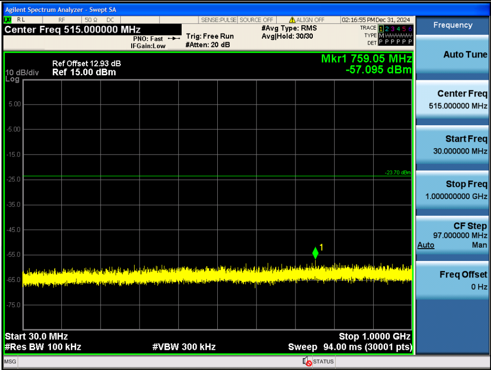
11G-Ant1-2462-30~1000-PASS
