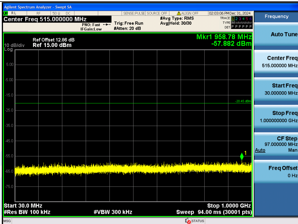
11G-Ant1-2412-30~1000-PASS
