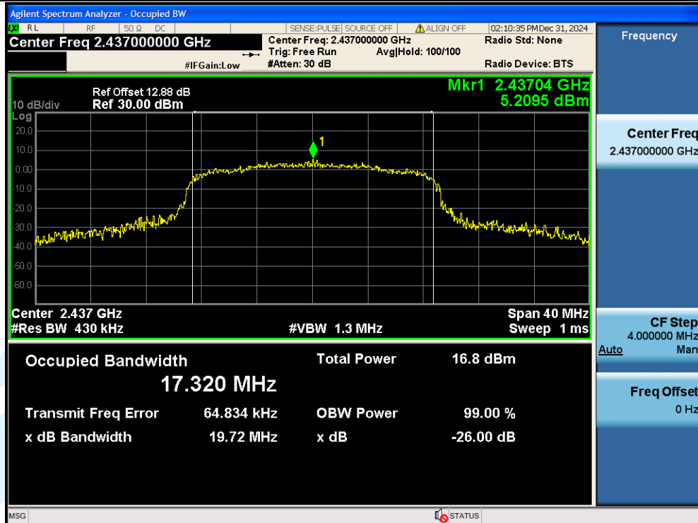
11G-Ant1-2437
