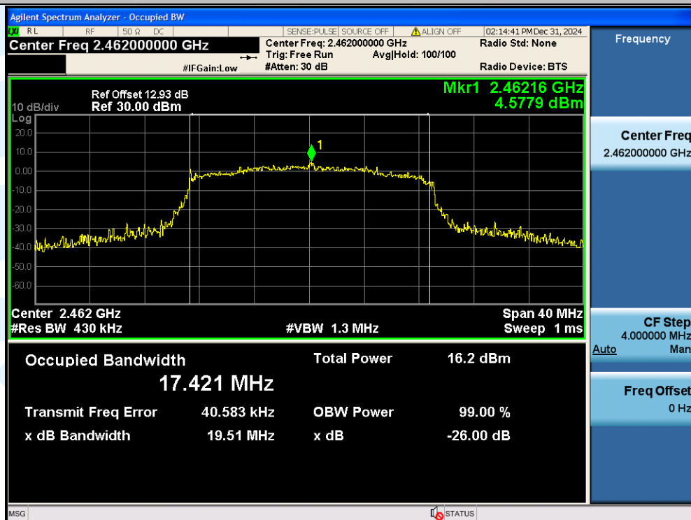
11G-Ant1-2462
