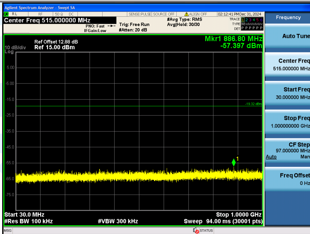
11G-Ant1-2437-30~1000-PASS
