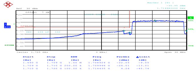
10MHz_Low_QPSK_50@0 99.00dBm
