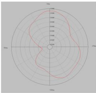
E2 plane
