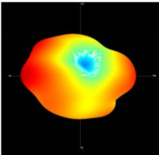
E1 plane
