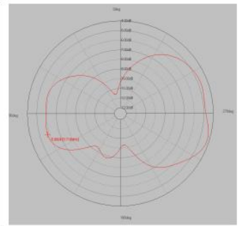
E2 plane
