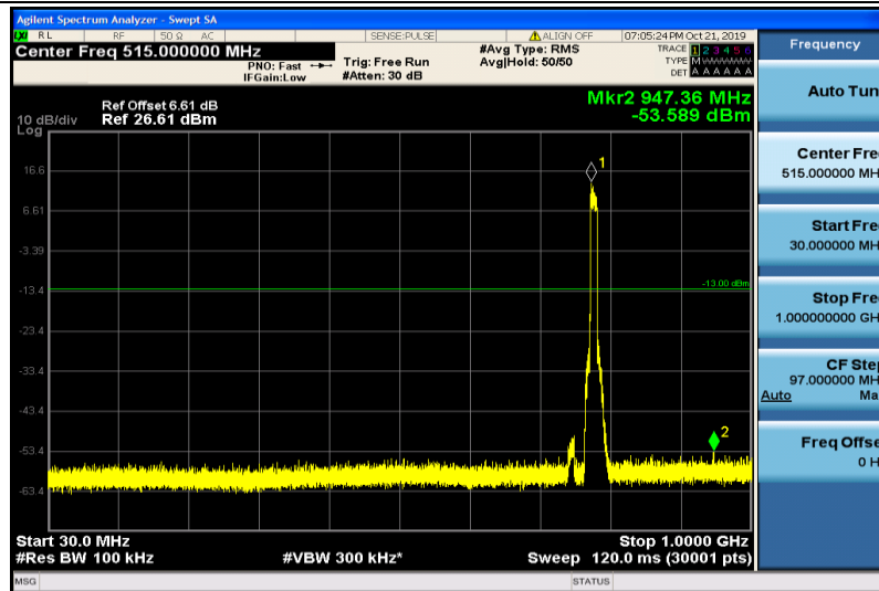
Band13-10MHz-QPSK-23230-50RB#0-30~1000MHz
