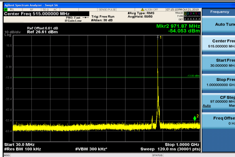
Band13-5MHz-QPSK-23230-1RB#0-30~1000MHz
