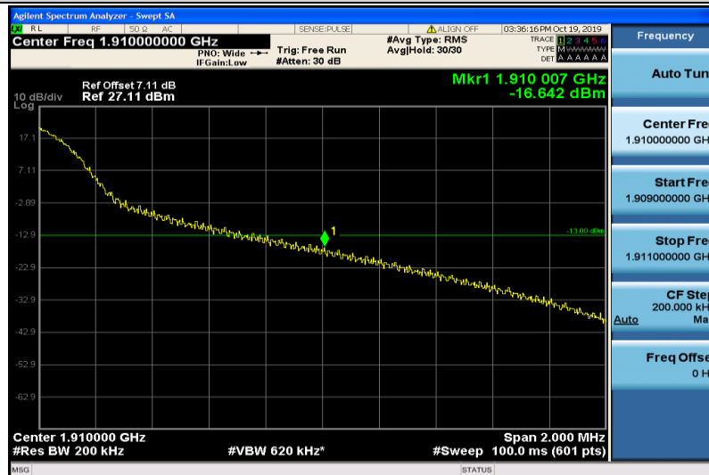
Band2-20MHz-16QAM-19100-1RB#99
