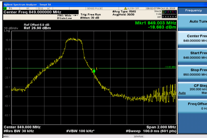
Band5-3MHz-QPSK-20635-1RB#14
