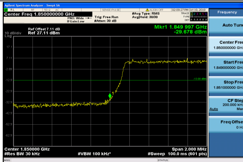
Band2-3MHz-16QAM-18615-15RB#0
