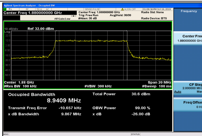
Band2-10MHz-QPSK-18900-50RB#0-8.9409
