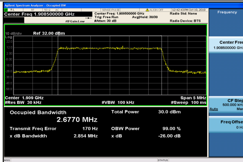
Band2-3MHz-QPSK-19185-15RB#0-2.6770
