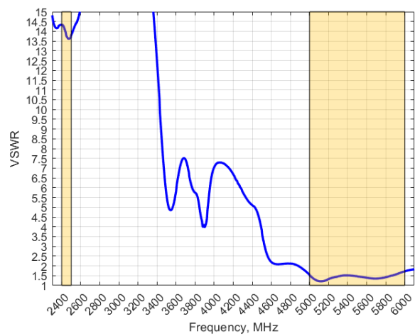
VSWR
