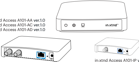
in:xtnd Access A101-IP ver.1.0
