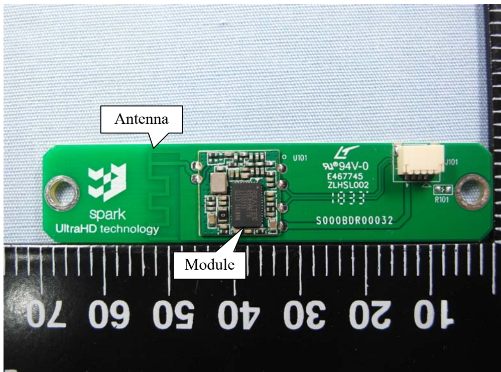
(30) EUT Photo
