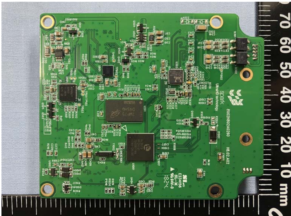
(24) EUT Photo
