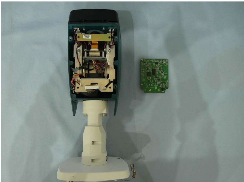
(20) EUT Photo
