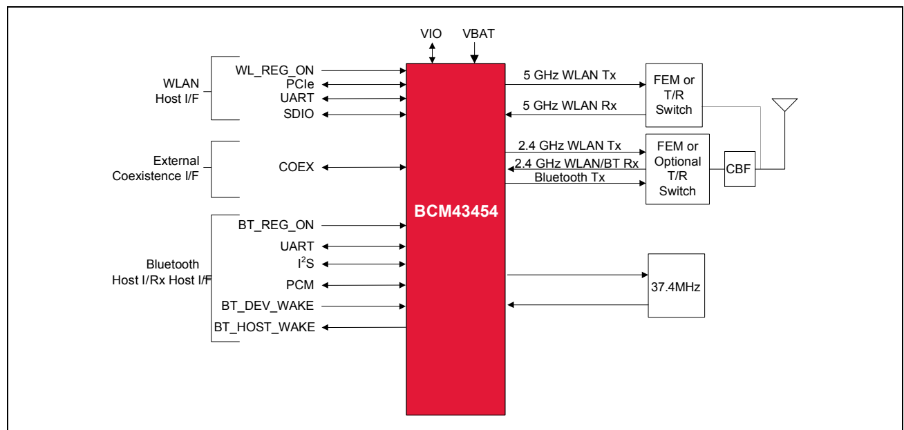
Bluetooth/Wifi module Block Diagram
