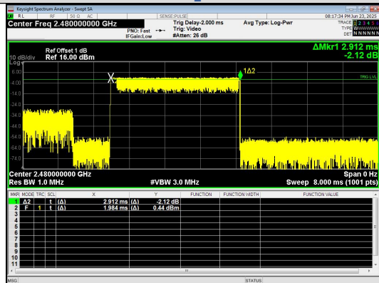
Pulse Width \pi/4 QPSK_2-DH5
