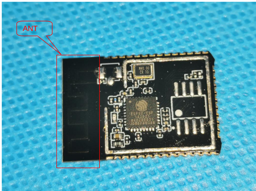
Photo 6 - ESP-C3-32S
