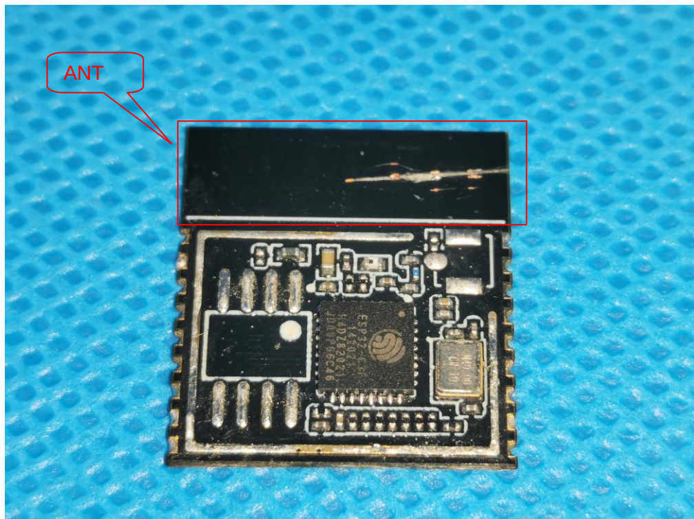
Photo 4 - ESP-C3-13
