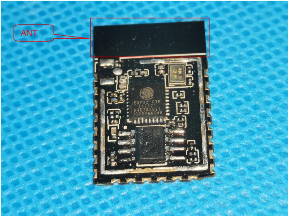
Photo 2 - ESP-C3-12F
