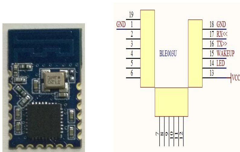
BLE003U Module
