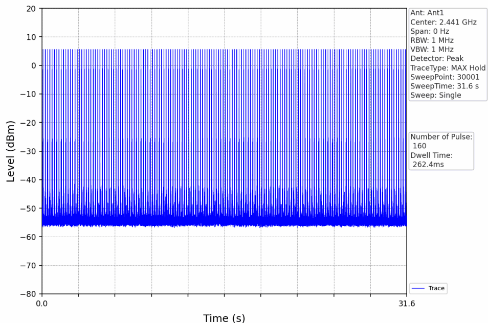
8DPSK_3DH3_HOPP_Ant1_NTNV
