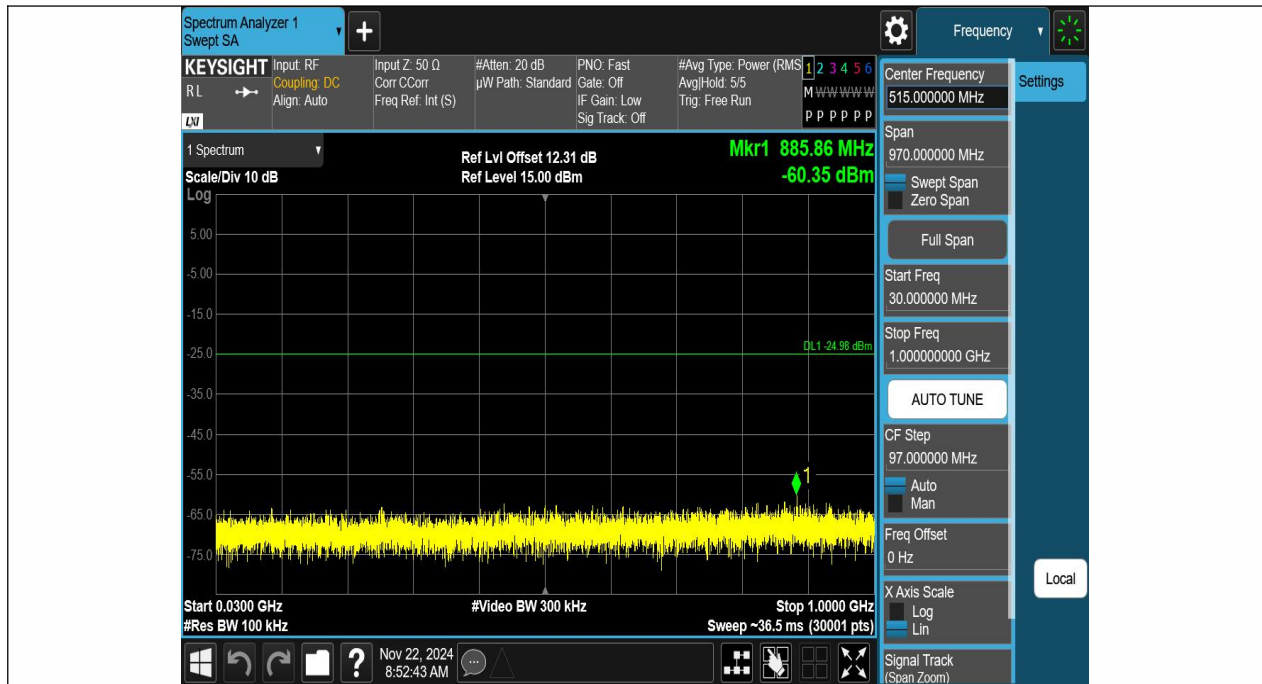
BLE_2M-Ant1-2402-30~1000-PASS
