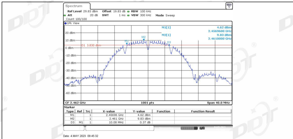
11B Ant2 2462
