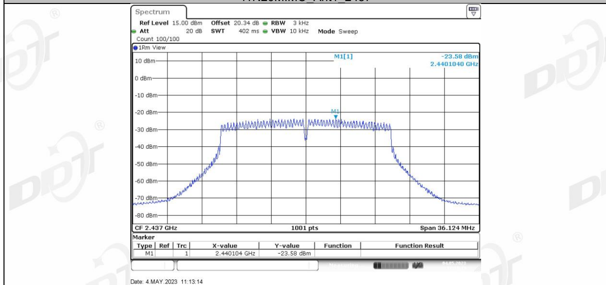
11N20MIMO Ant2 2437
