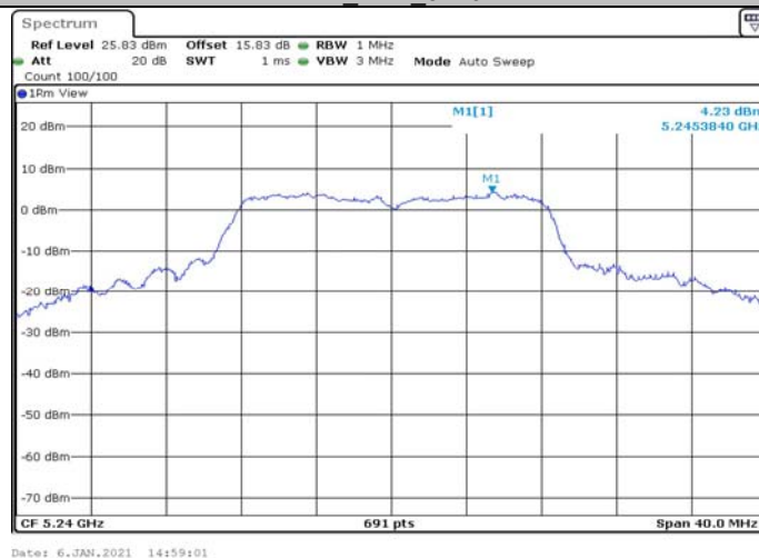
11A_Ant1_5240
