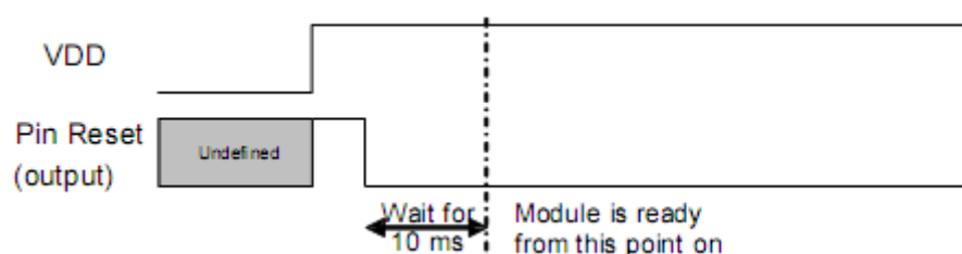
Figure 38. POR Timing Diagram
