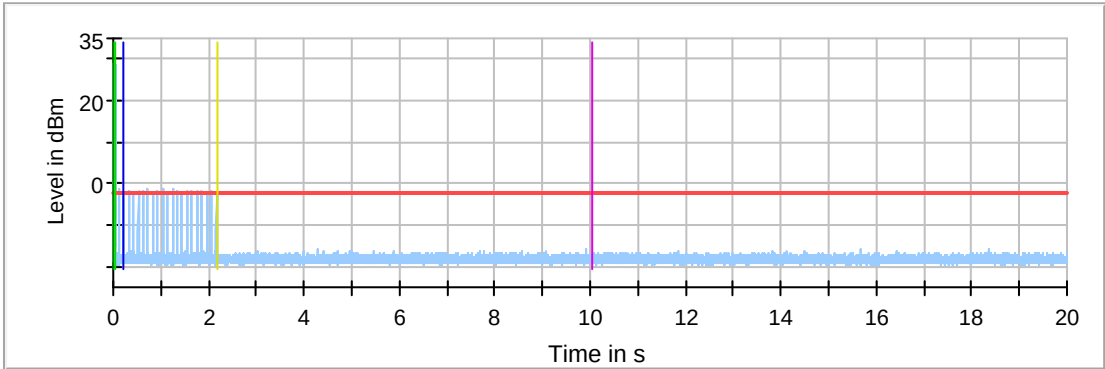
802.11ac VHT80 5530MHz
