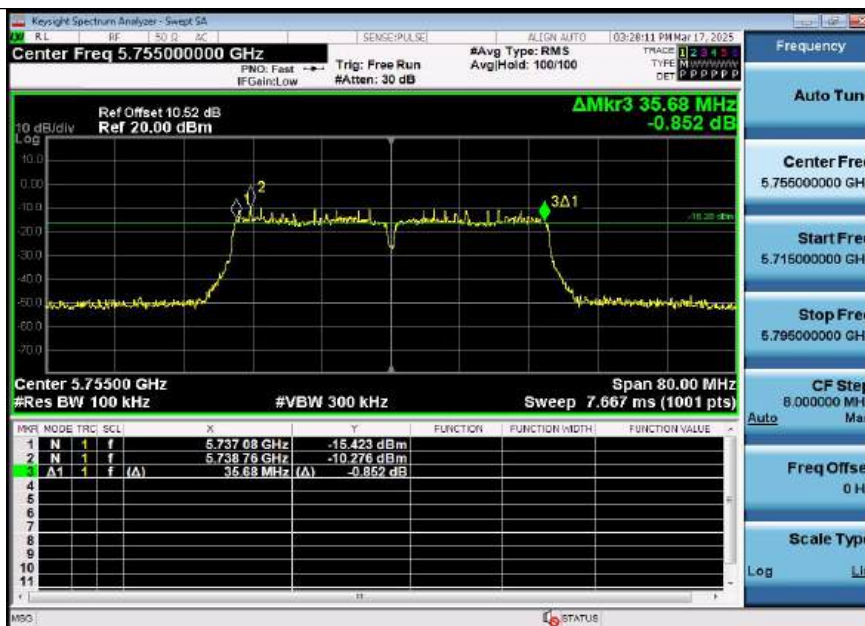
11N40SISO-Ant1-5755-PASS
