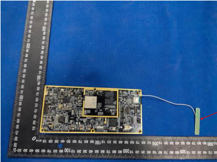
BT&WIFI Antenna
