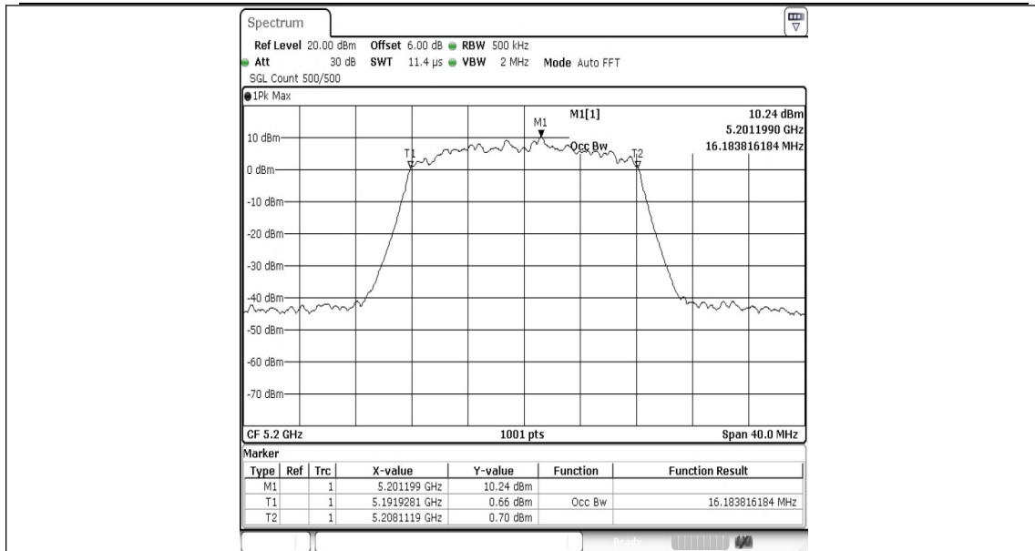
11A-Ant1-5200
