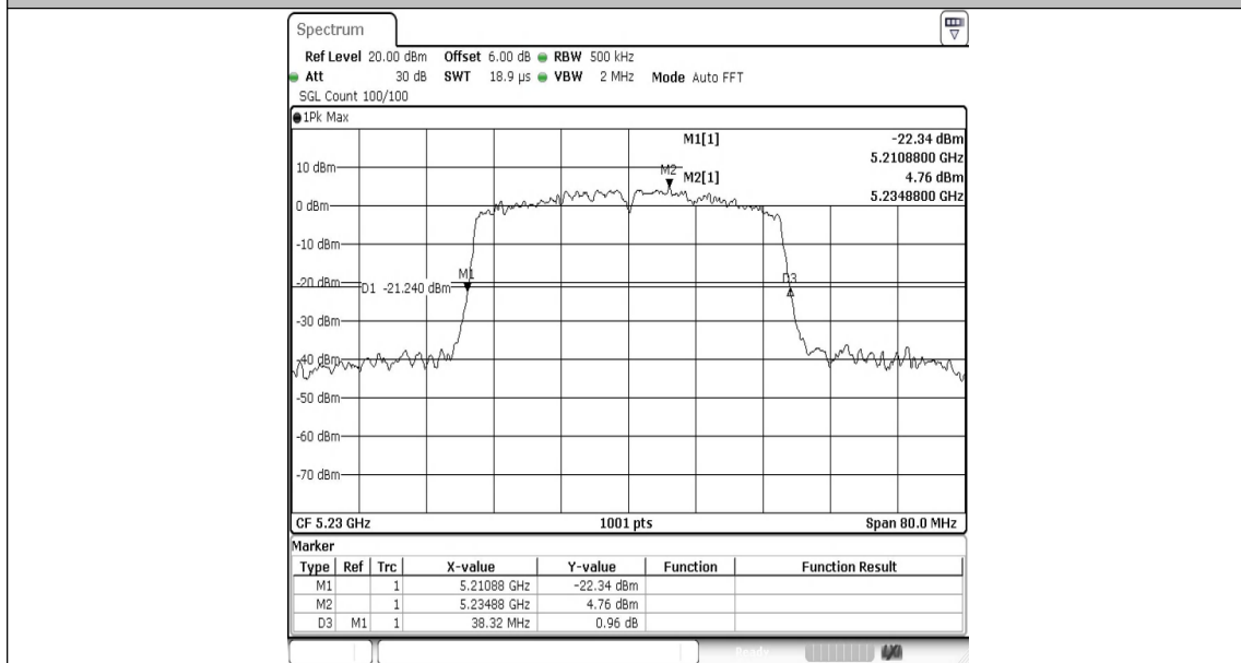
11AC40MIMO-Ant1-5230
