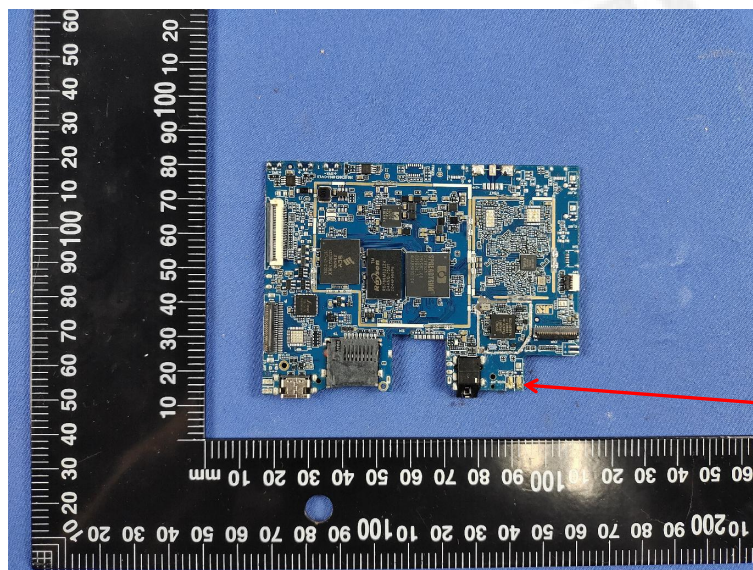
Bluetooth/WiFi Antenna
