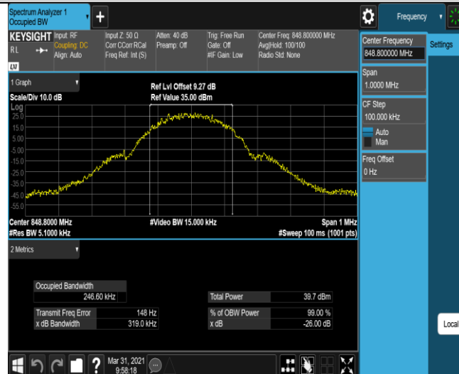
GSM850-251-3-0.3190
