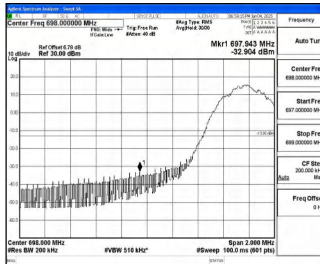
Band85-10MHz-QPSK-134052-1-0-Low--32.90-PASS
