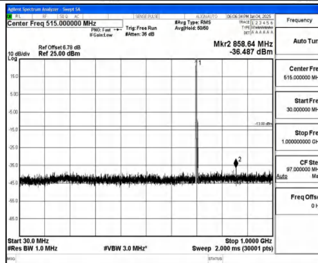
Band85-5MHz-QPSK-134092-1-0-Low-30-1000--36.49-PASS
