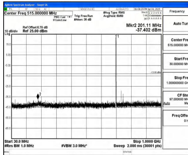
Band85-5MHz-16QAM-134092-1-0-Low-30-1000--37.4-PASS
