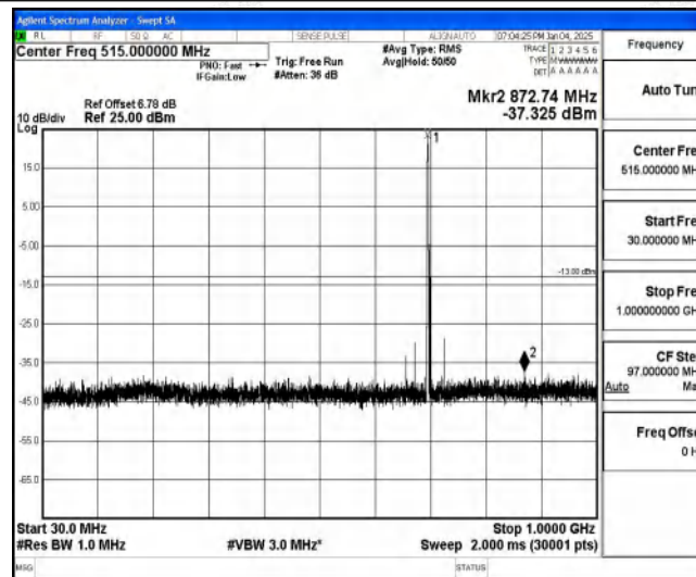
Band85-10MHz-QPSK-134092-1-0-Low-30-1000--37.33-PASS
