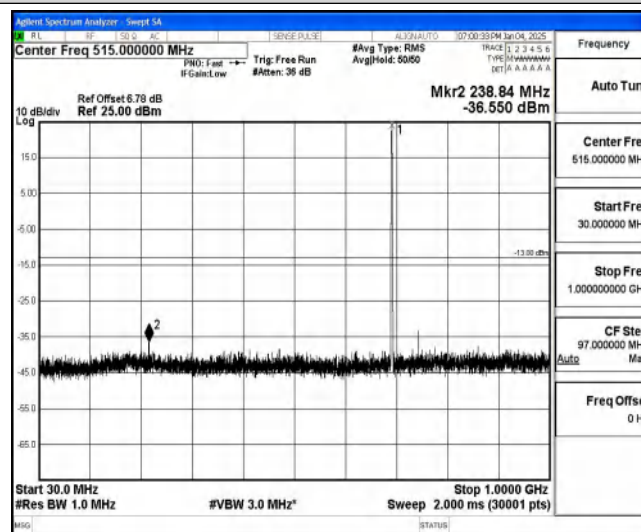
Band85-10MHz-QPSK-134052-1-0-Low-30-1000--36.55-PASS
