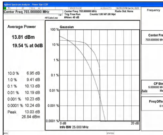
Band85-10MHz-QPSK-134052-1-0-Low-10.13-&lt;=13-PASS
