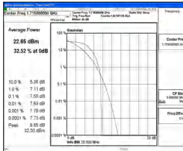
Band4-10MHz-QPSK-20000-1-0-Low-7.55-13-PASS
