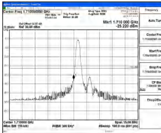
Band4-5MHz-16QAM-19975-1-0-Low--25.22-PASS
