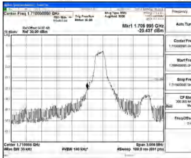
Band4-1.4MHz-16QAM-19957-1-0-Low--20.44-PASS
