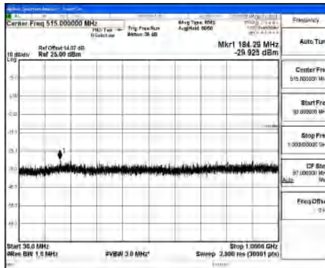
Band4-20MHz-QPSK-20050-1-0-Low-30-1000--29.93-PASS
