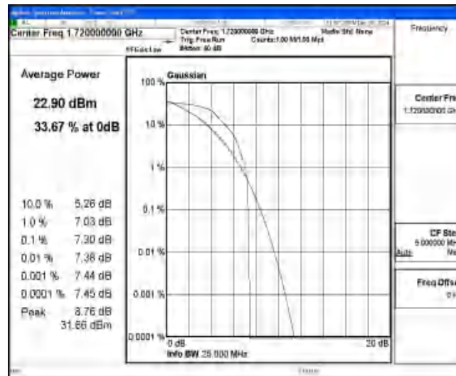
Band4-20MHz-QPSK-20050-1-0-Low-7.30-&lt;=13-PASS
