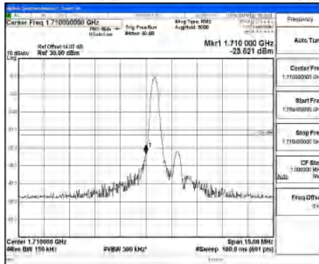
Band4-5MHz-QPSK-19975-1-0-Low--23.62-PASS
