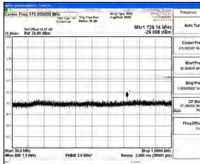
Band4-10MHz-QPSK-20000-1-0-Low-30-1000--29.7-PASS
