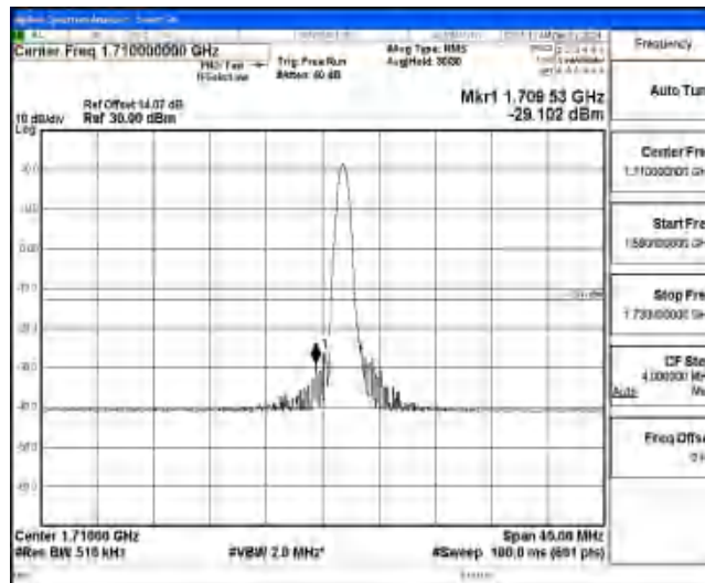
Band4-20MHz-16QAM-20050-1-0-Low--29.10-PASS
