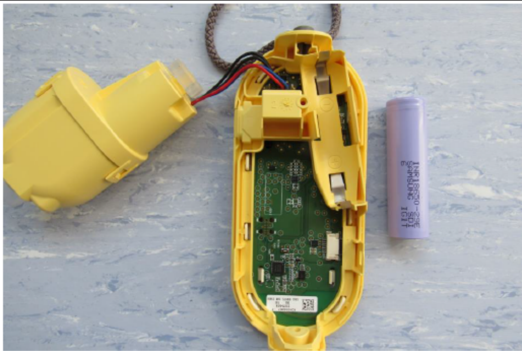
EUT PCB TOP I
