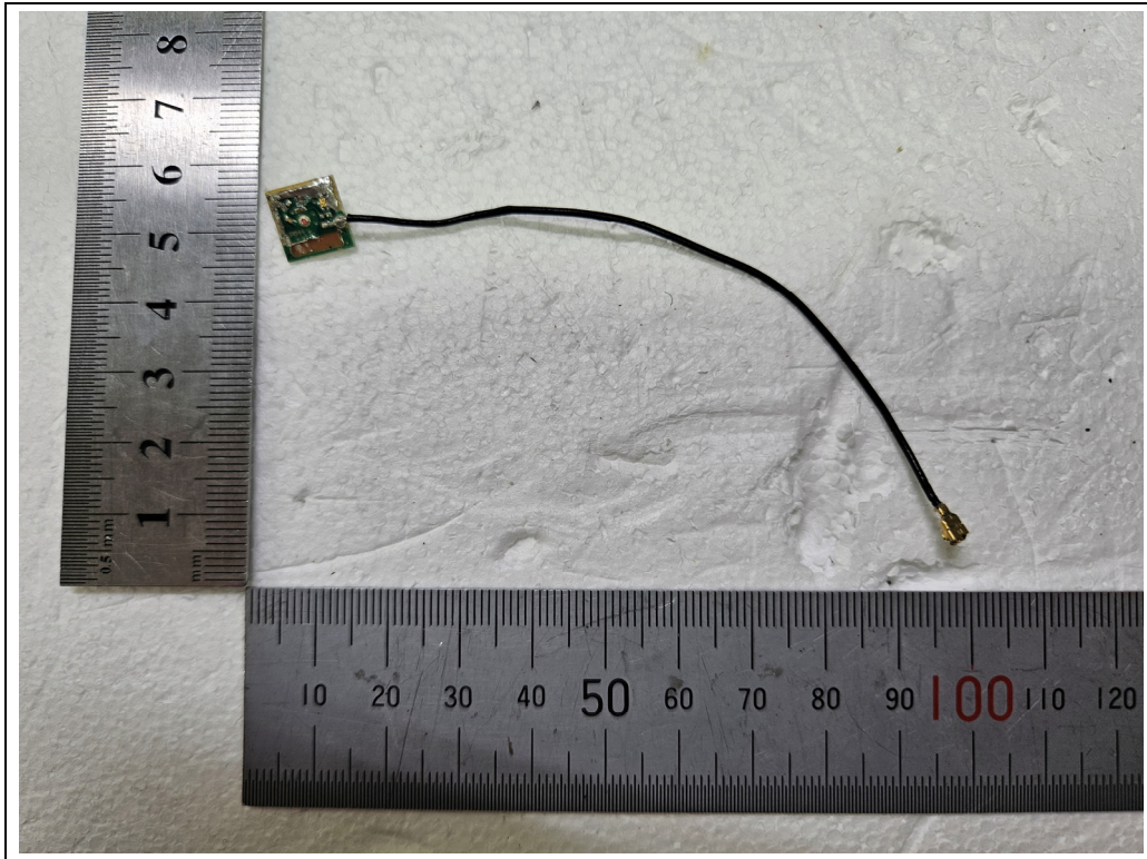
<GNSS Antenna>
