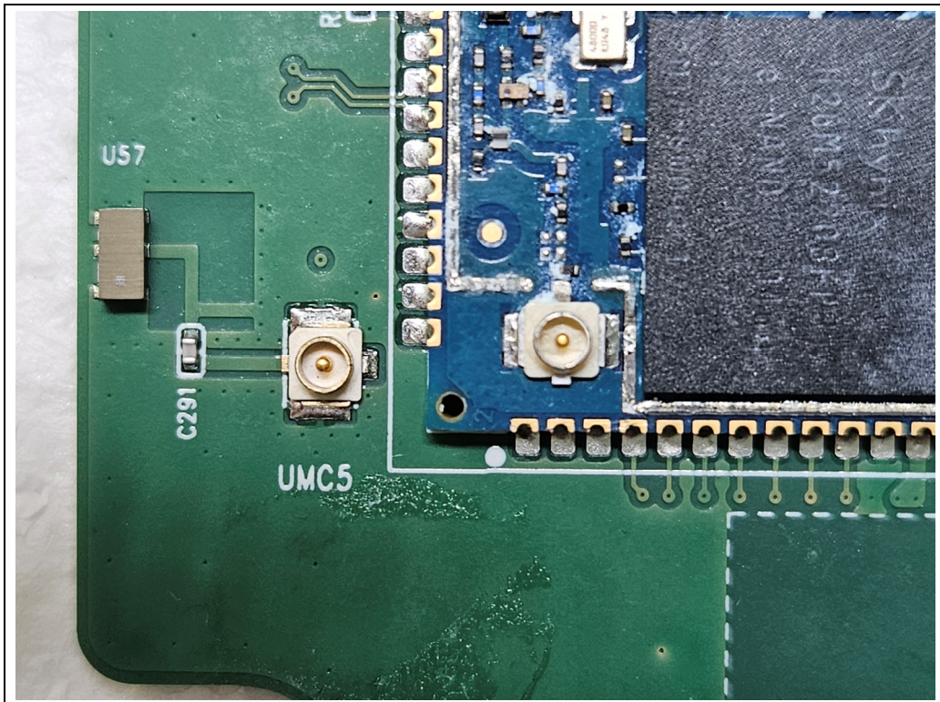
<WLAN Antenna>
