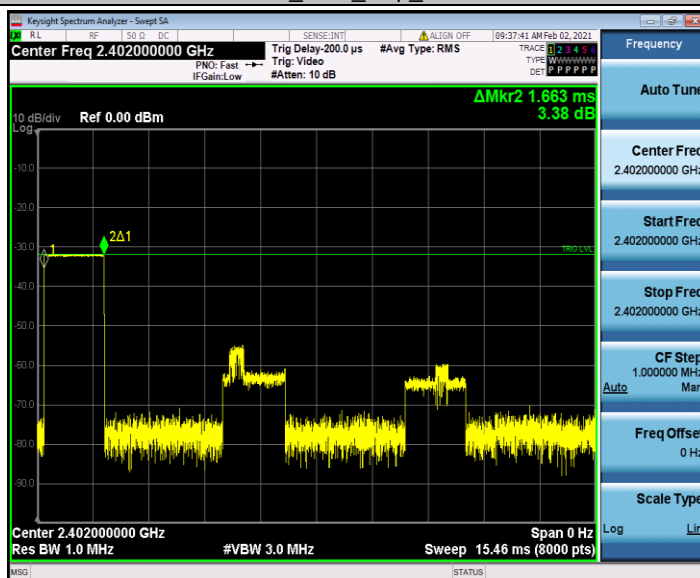
DH3_Ant1_Hop_2402
