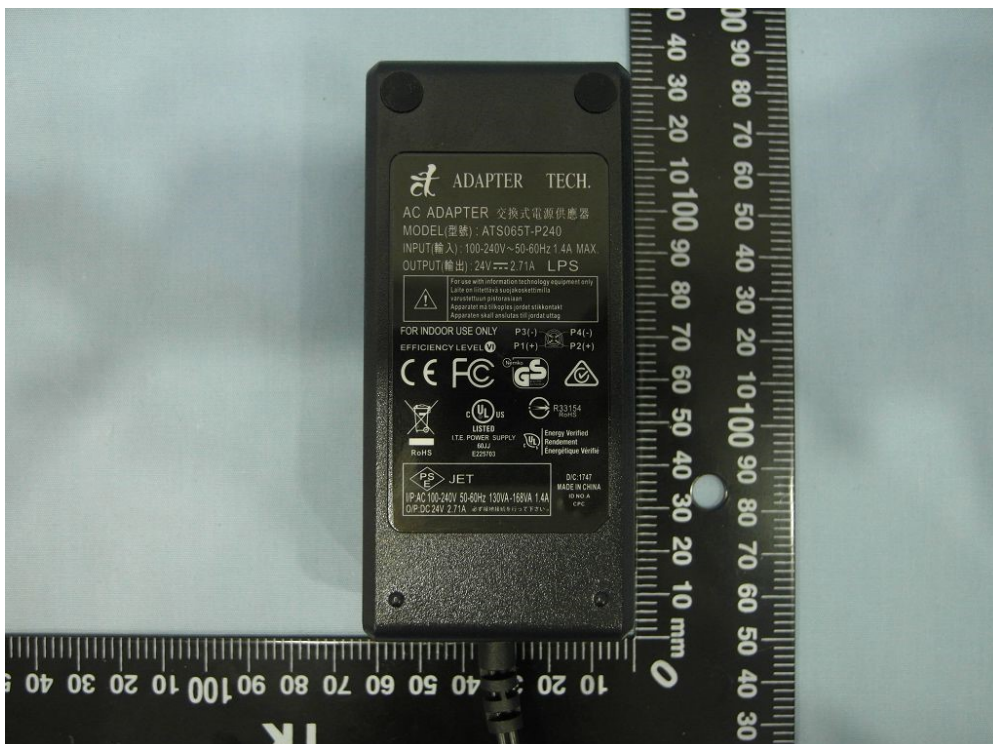
(53) EUT Photo
