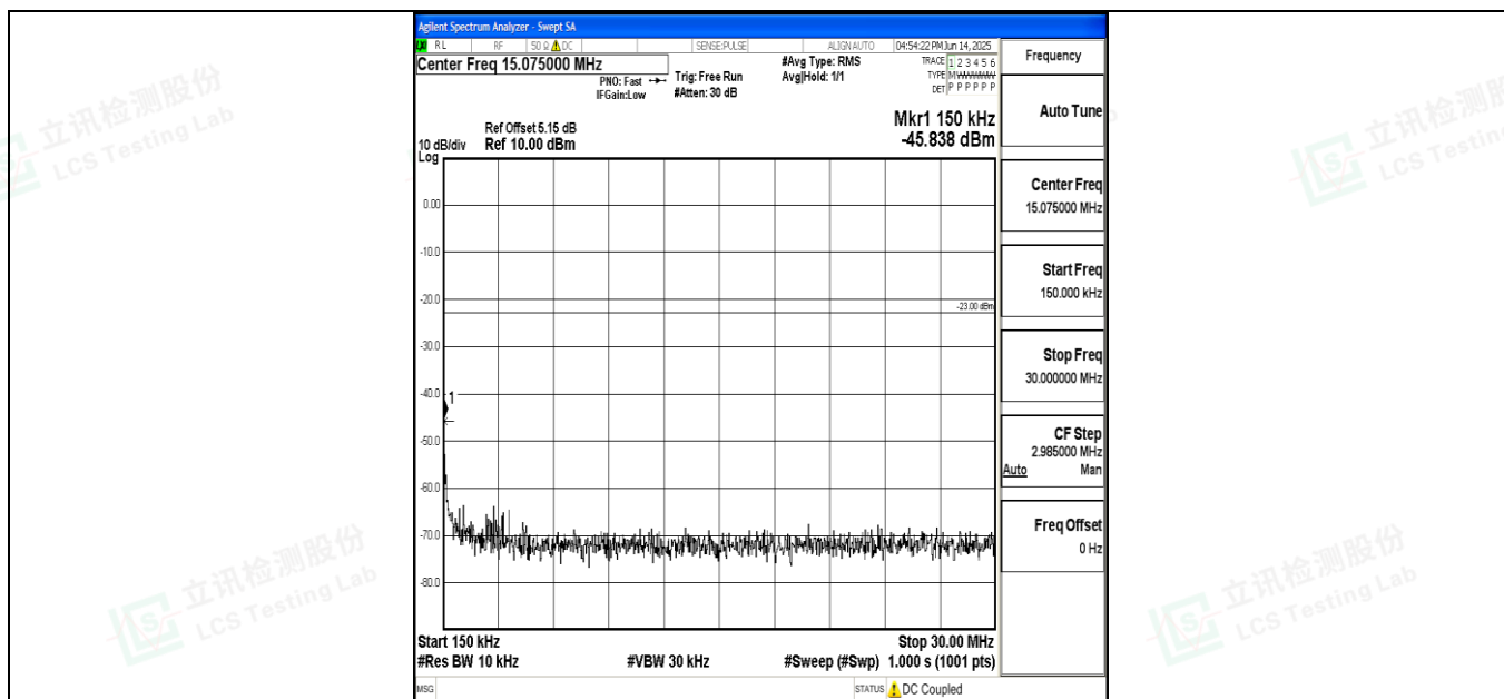
Band71 20MHz 16QAM 133372 1RB#0 0.15~30 0.15~30
