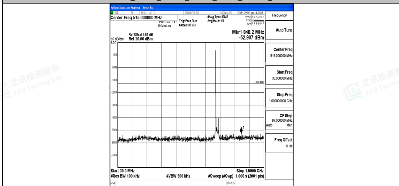
Band71 20MHz 16QAM 133372 1RB#0 30~1000 30~1000
