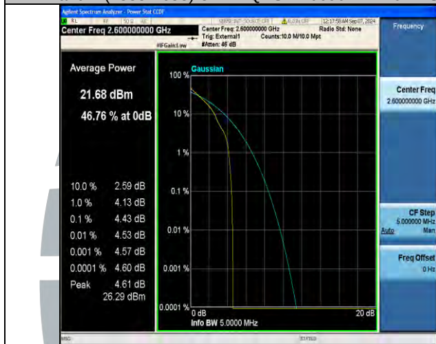
Band41(2555-2655)-5MHz-QPSK-41215-1RB#0-PASS
