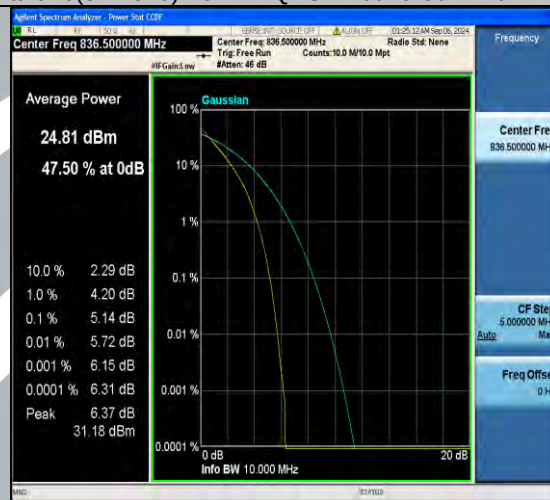
Band26(824-849)-10MHz-QPSK-26990-50RB#0-PASS
