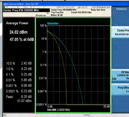
Band26(824-849)-3MHz-QPSK-27025-15RB#0-PASS
