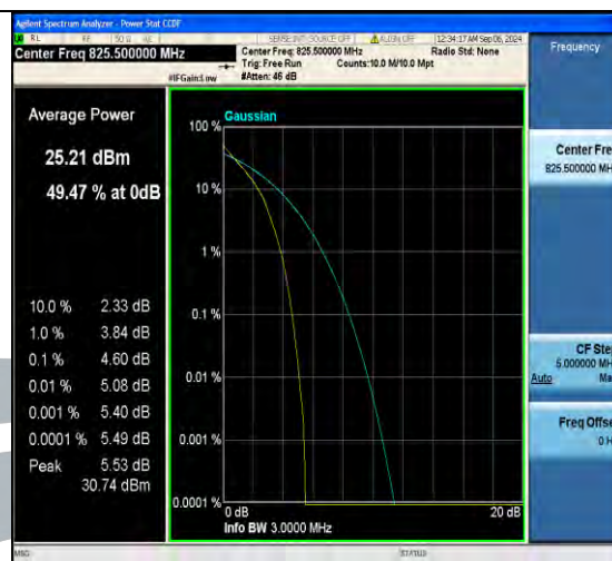
Band26(824-849)-3MHz-QPSK-26915-15RB#0-PASS
