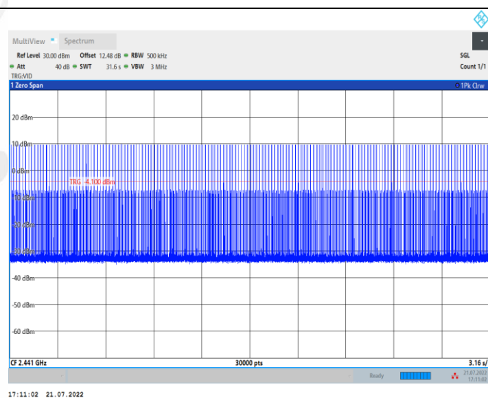
2DH3_Ant1_Hop
