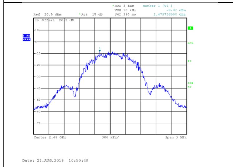
Figure 27. 2480.0 MHz, BLE
